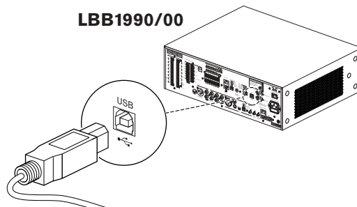
Рисунок 3.5 Подключение к контроллеру LBB 1990/00
