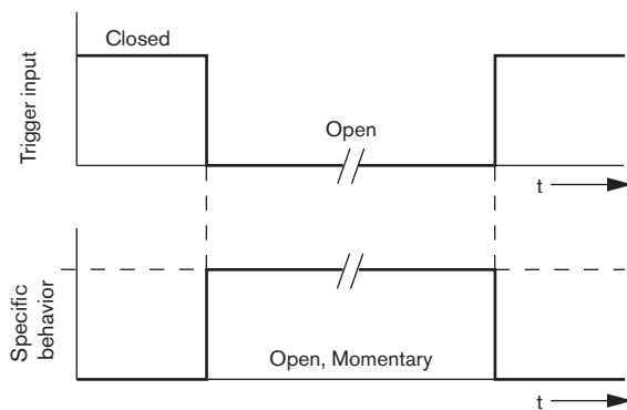
Рисунок 4.39 Открыть, Кратковременно
