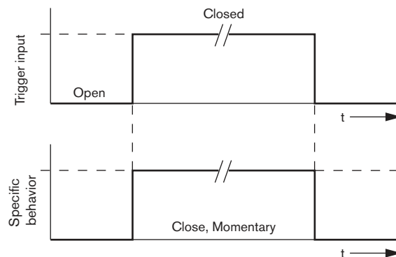
Рисунок 4.38 Закреть, Кратковременно
