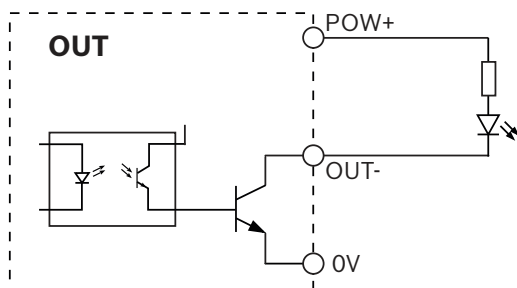
Функциональные возможности выхода "открытый коллектор"
