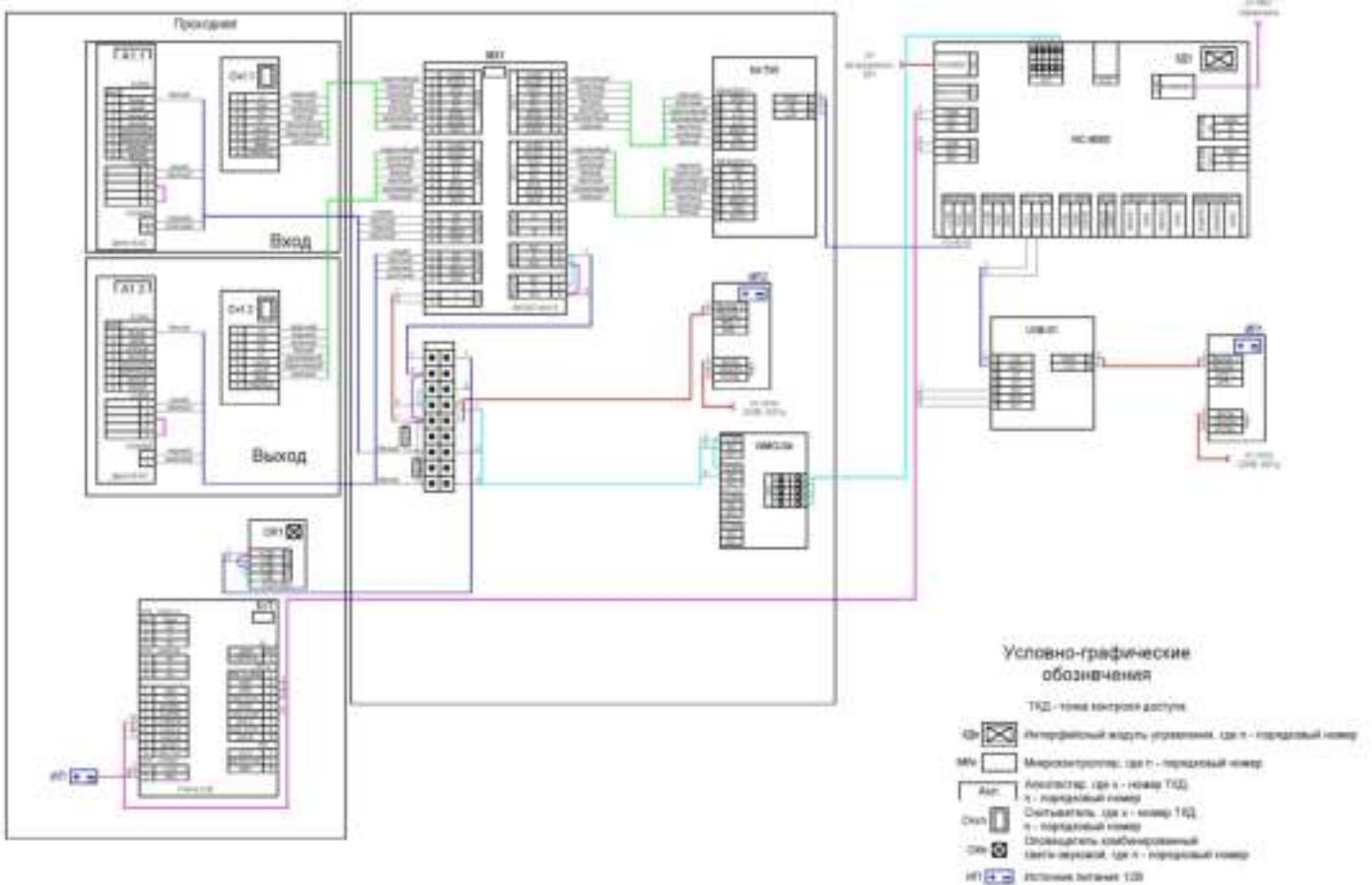
Схема подключения платы GHOST к оборудованию Рarves
