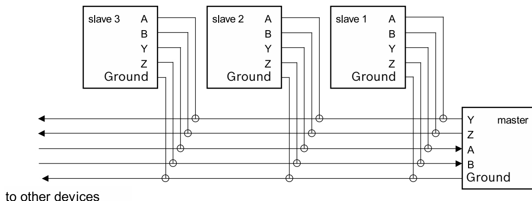
Рис. 5.3: Структура сети RS-485
