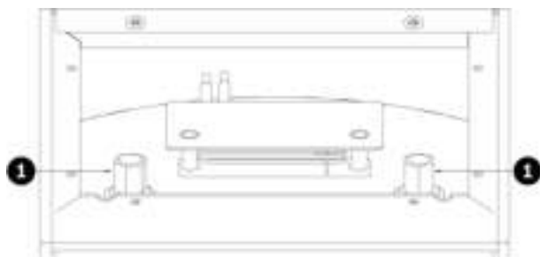
Рис. 4.4: Доступ к фиксирующим болтам
