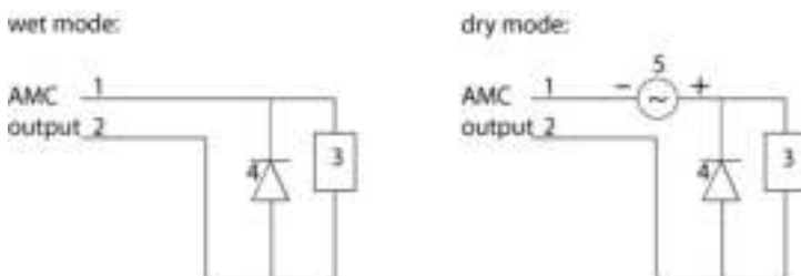
Рис. 4.13: Схема восстановительных диодов
