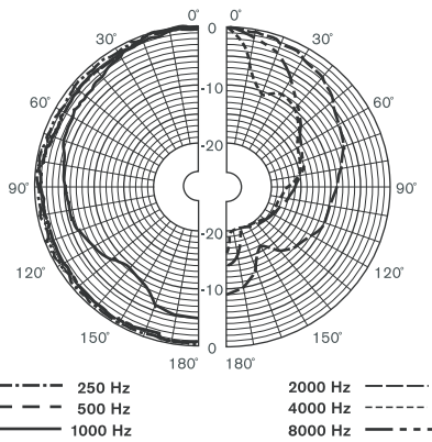
Полярная диаграмма (для розового шума)
