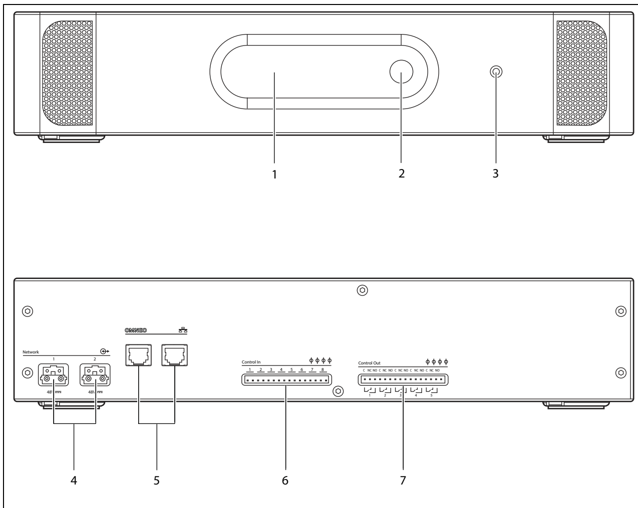
рисунок 8.2: Вид интерфейса OMNEO спереди и сзади
