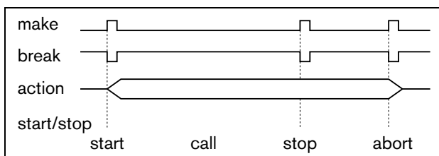
рисунок 48.9: Переключение с завершением фазы и прерыванием при повторном нажатии (2)
