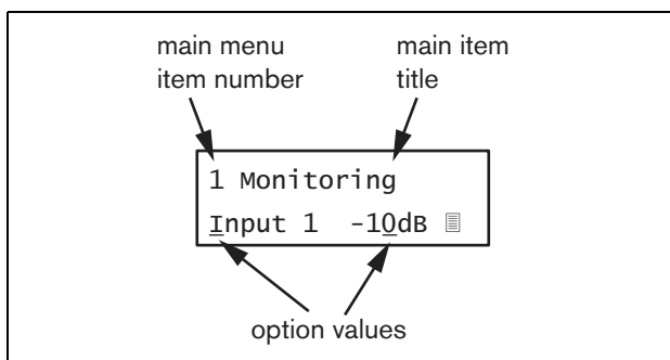
рисунок 8.9: Элементы экрана пункта меню
