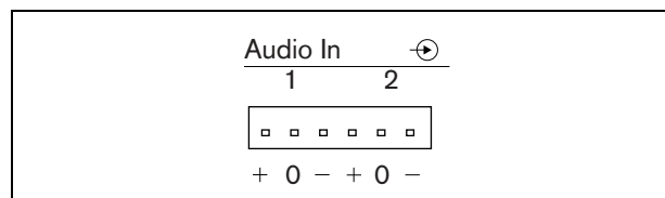
рисунок 9.10: Разъемы аудиовходов
