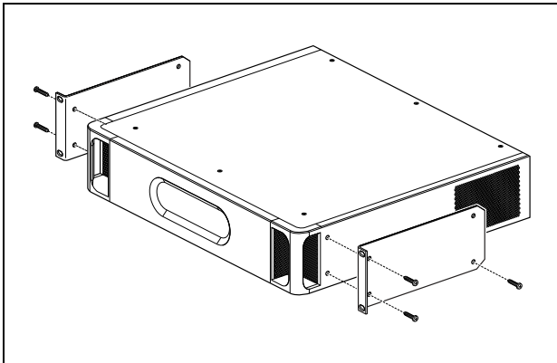
рисунок 11.17: Установка
