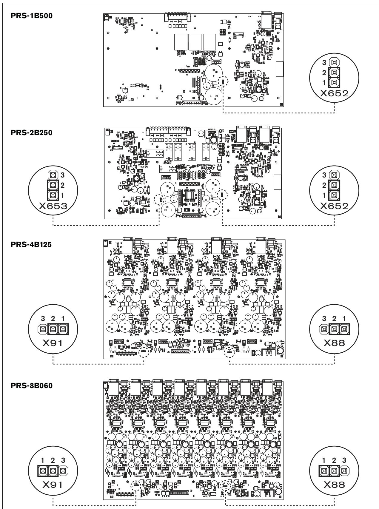
рисунок 11.16: Вид верху выходных плат с перемычками для управления вентиляторами
