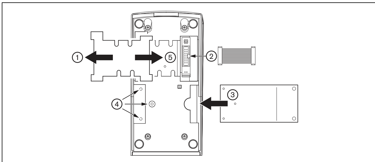
рисунок 17.5: Установка
