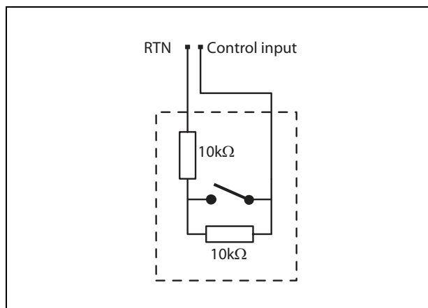
рисунок 19.6: Контролируемый вход управляющего сигнала
