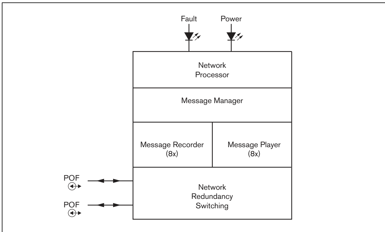
рисунок 24.1: Блок-схема
