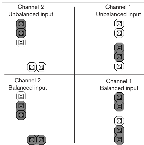
рисунок 11.14: Установка переключек
