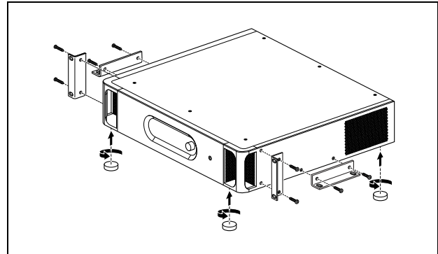
рисунок 7.6: Установка
