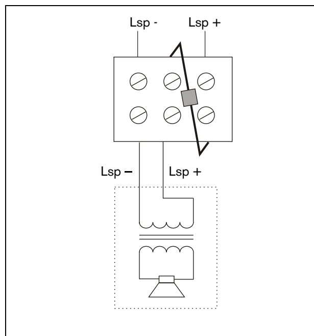
рисунок 15.2: Принципиальная электрическая схема
