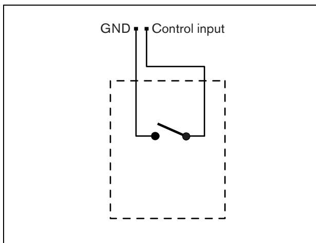
рисунок 21.7: Неконтролируемый вход управляющего сигнала
