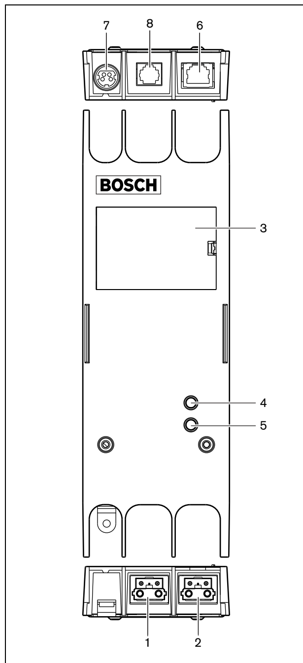
рисунок 23.2: Наружная сторона
