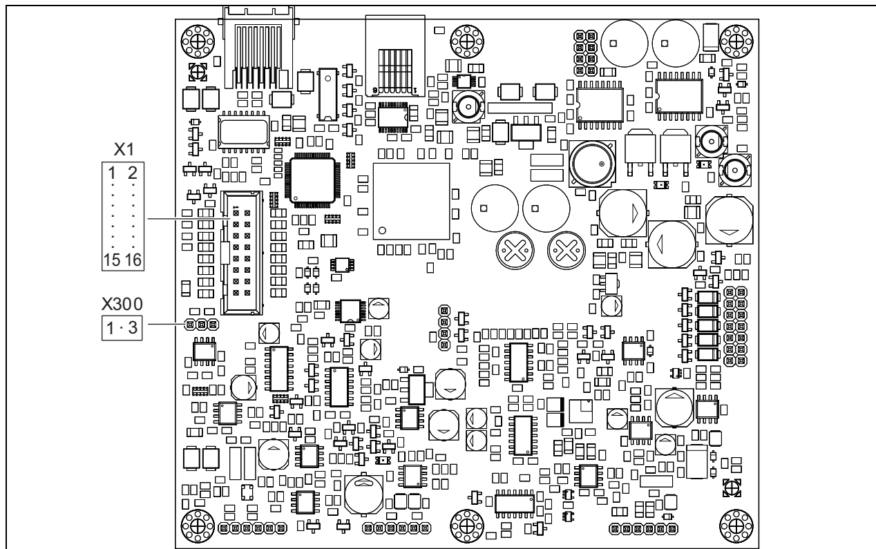
рисунок 22.13: Печатная плата PRS-CSRМ со стороны монтажа
