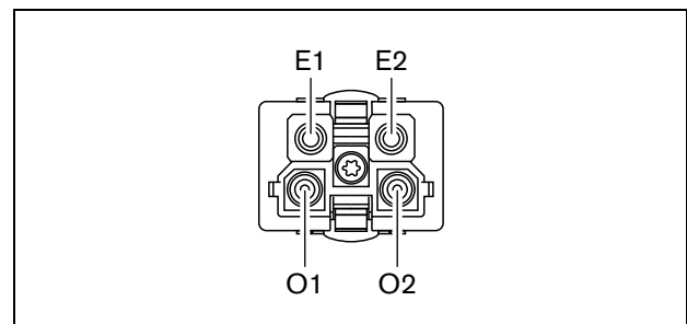
рисунок 30.26: Вид разъема спереди
