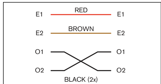
рисунок 30.27: Монтажная схема
