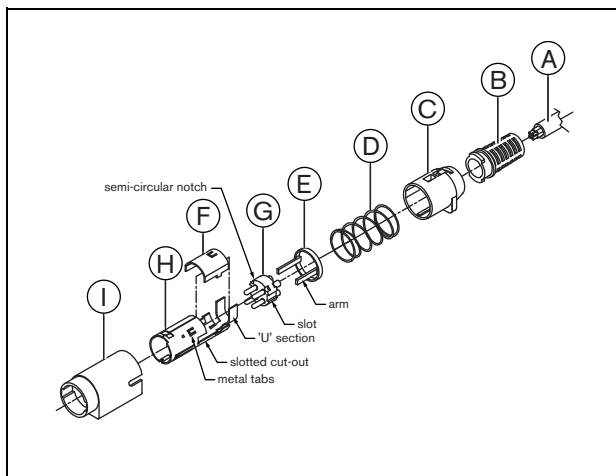
рисунок В.1: Сборочный чертеж
