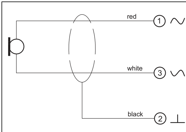
рисунок 22.5: Схема соединений LBB9082
