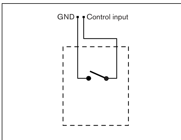
рисунок 23.8: Неконтролируемый вход управляющего сигнала
