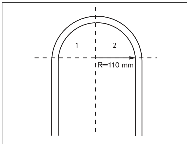
рисунок 32.7: Кривая U
