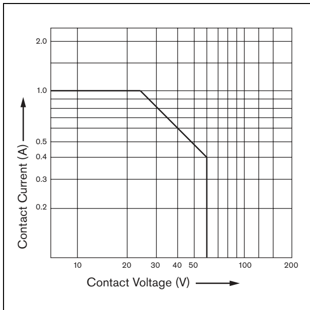
рисунки 5.16: Максимальная коммутируемая мощность
