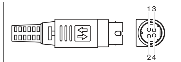
рисунок 26.6: Схема соединений (внешний вид)
