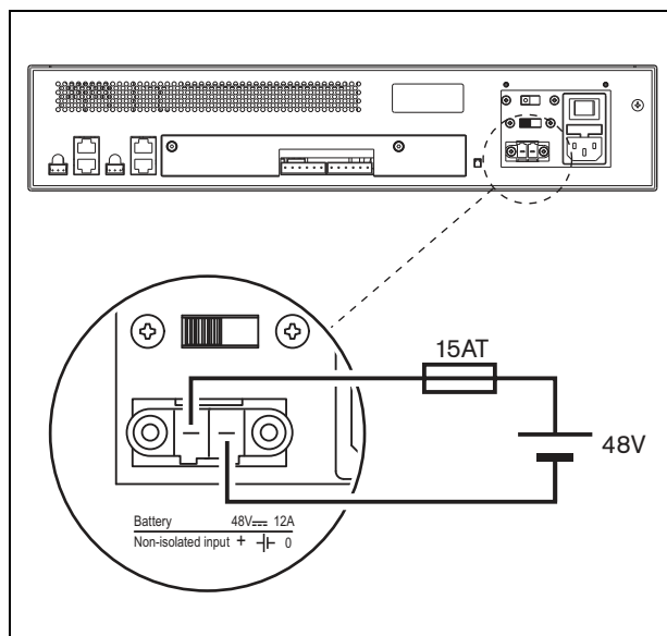
рисунок 11.15: Подключение резервного электропитания
