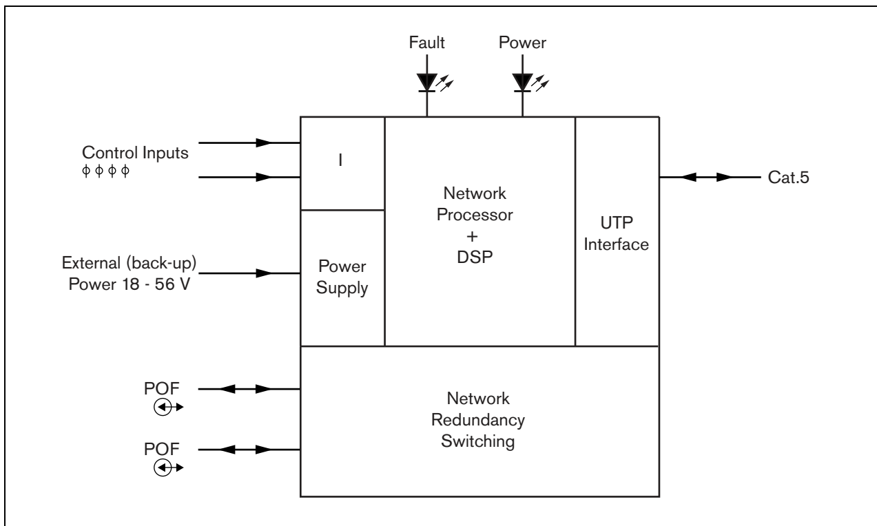
рисунок 23.1: Блок-схема
