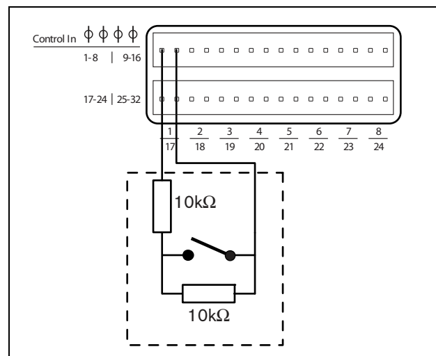
рисунок 10.6: Контролируемые входы управляющего сигнала с 1 по 8
