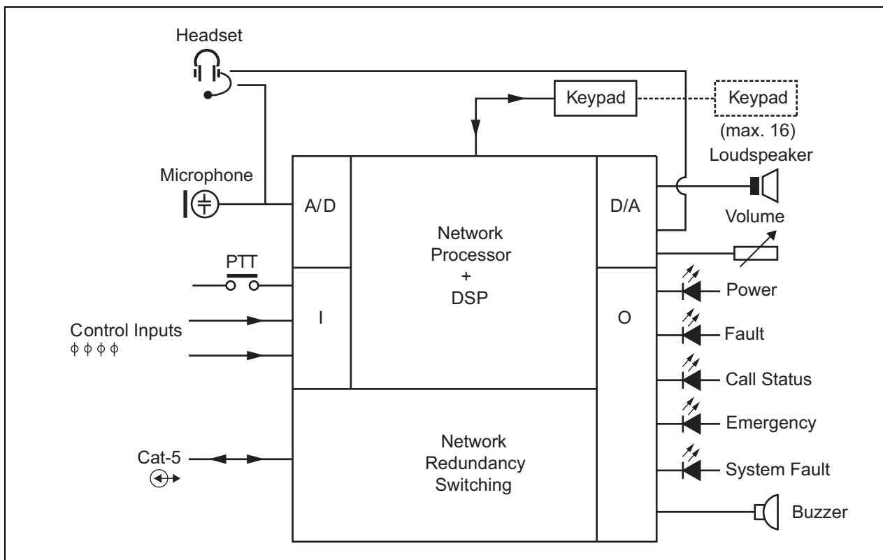
рисунок 22.1: Блок-схема PRS-CSRM
