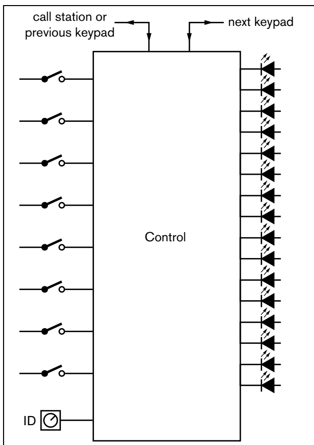
рисунок 17.1: Блок-схема
