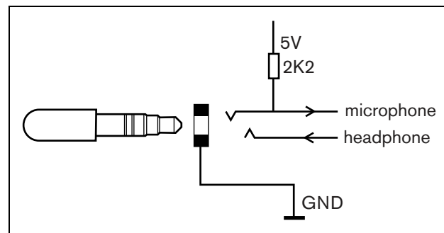
рисунок 16.2: Разъем гарнитуры
