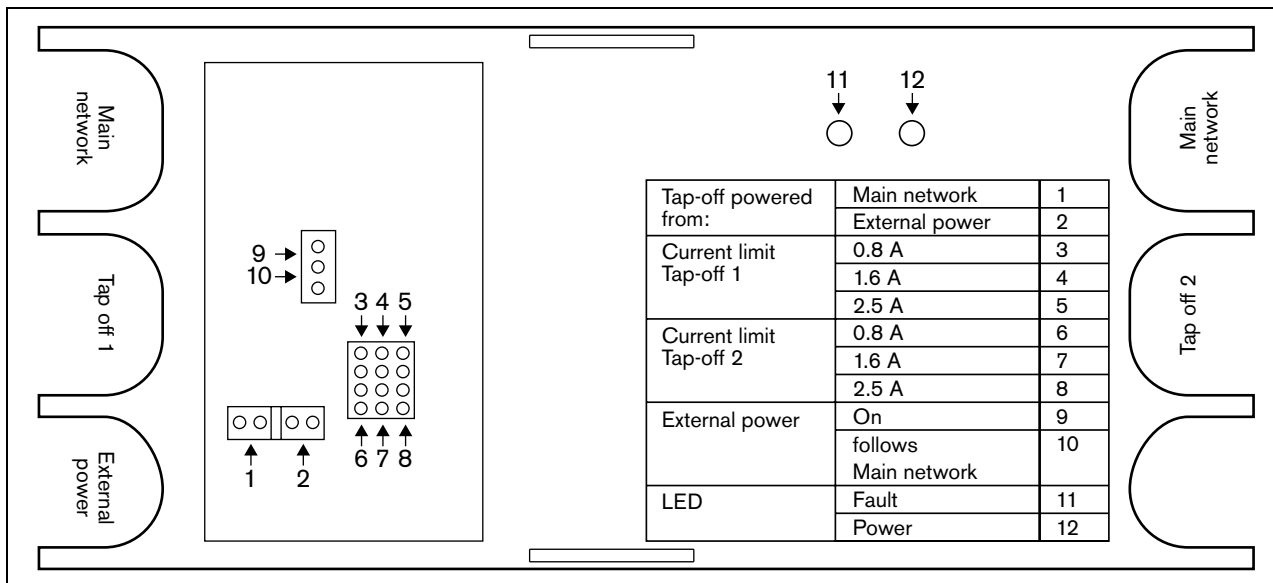
рисунок 26.4: Идентификация переключек
