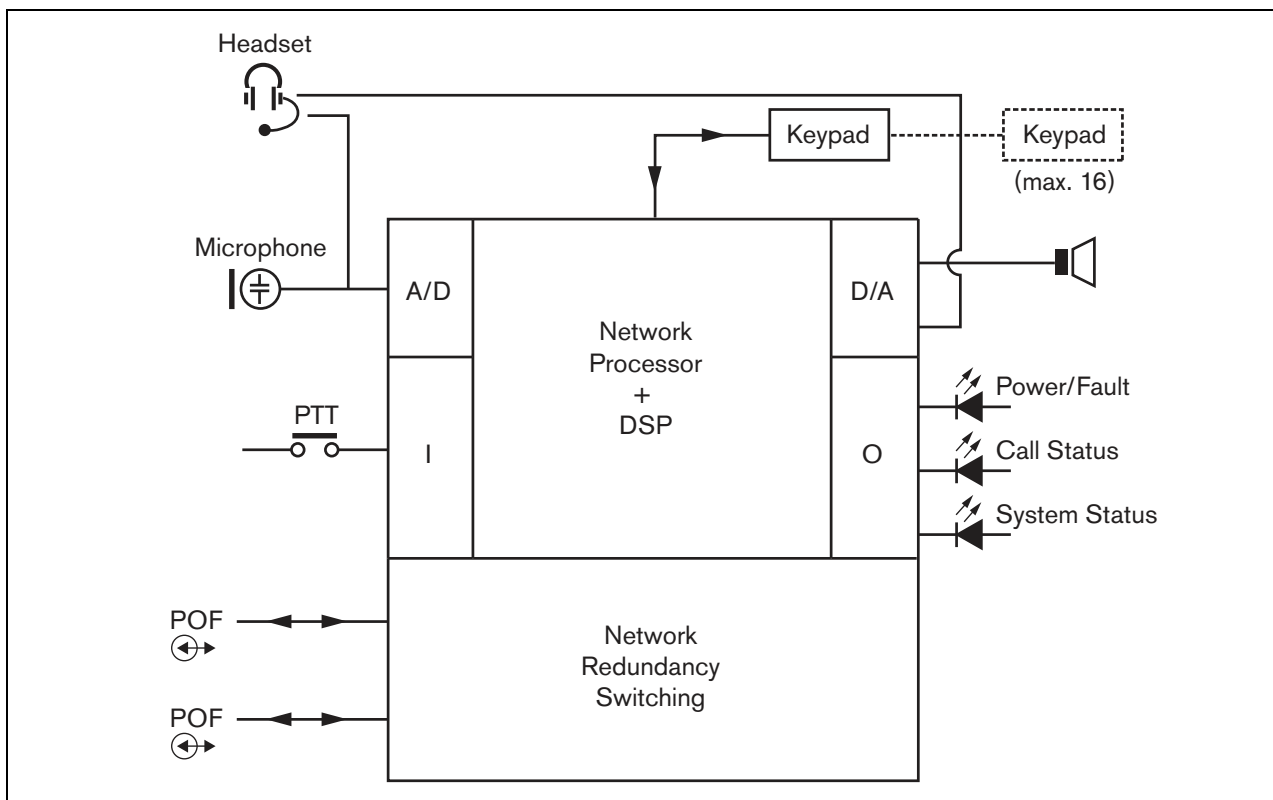
рисунок 16.1: Блок-схема
