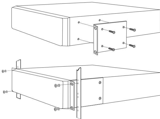
Рисунок 5.1: Монтаж 19-дюймовых кронштейнов и установка в стойку
