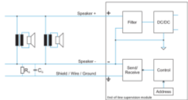
Принципиальная схема
