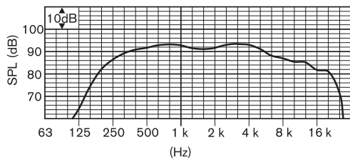
Частотная характеристика
