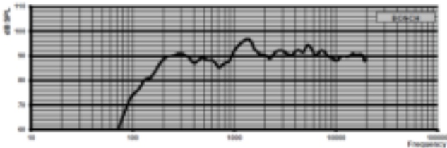
Частотная характеристика
