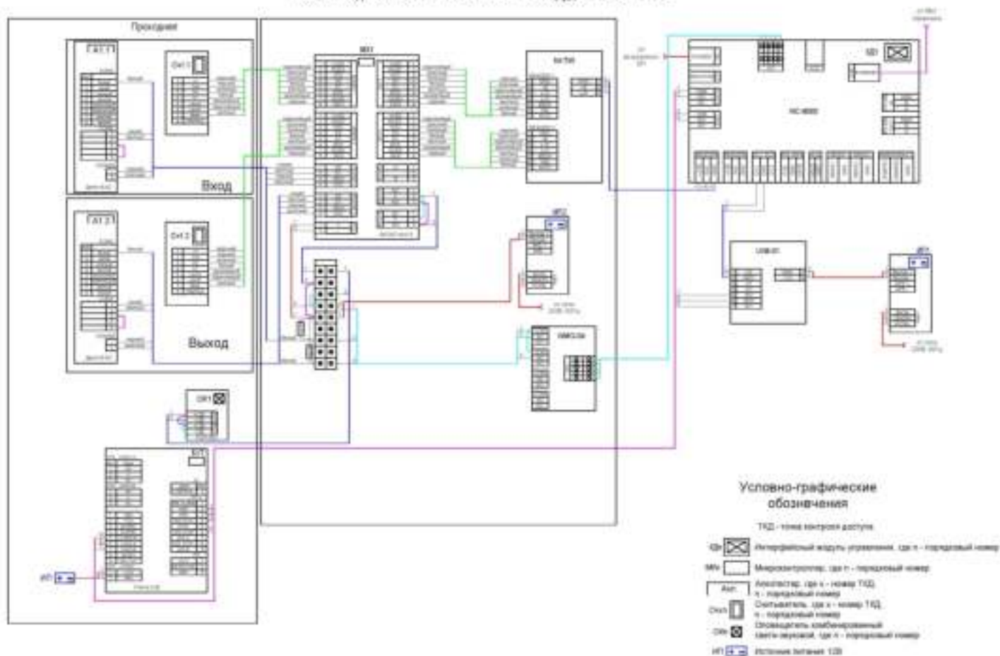
Схема подключения платы GHOST к оборудованию Parsec
