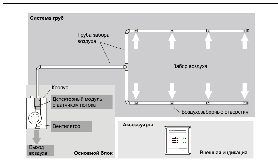
Рис. 2.1: Обзор дымовой аспирационной системы TITANUS®
