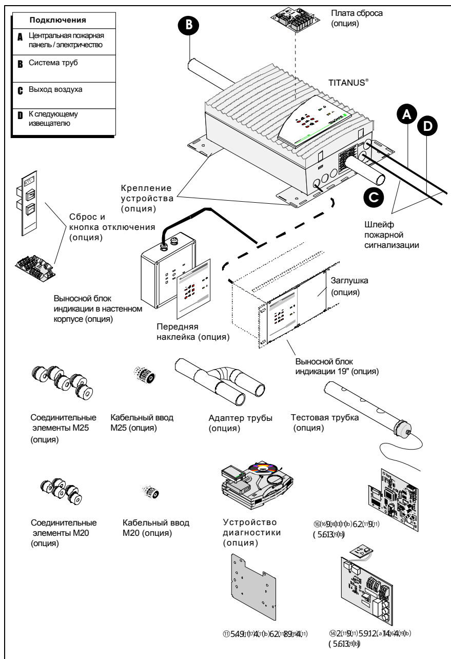
Рис. 2.3: Обзор TITANUS®
