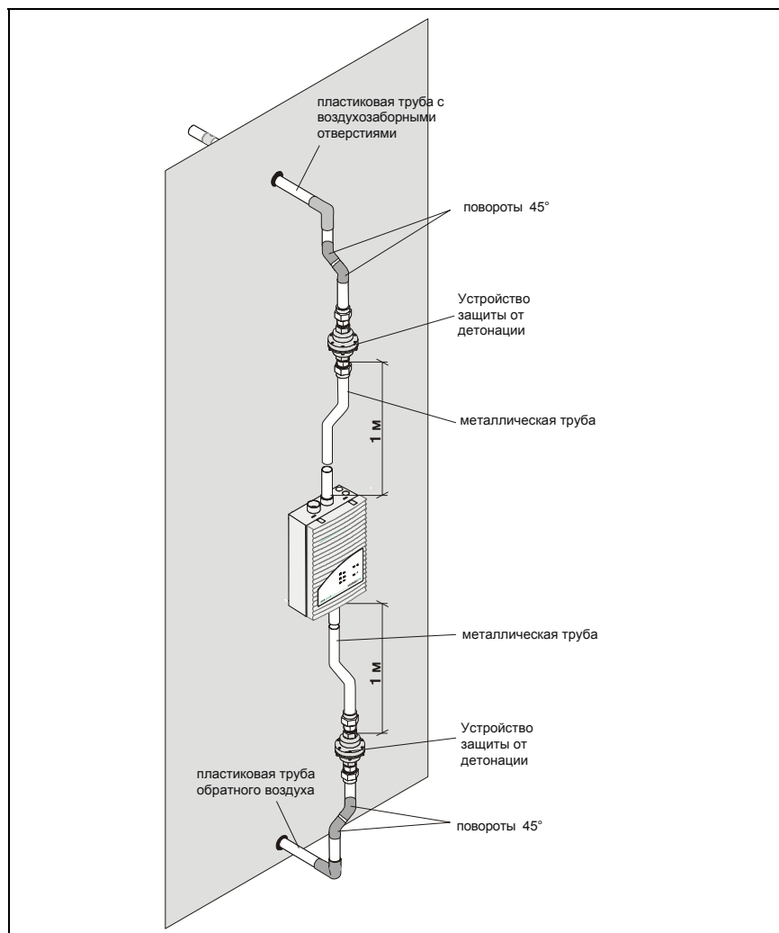
Рис. 6.13 Монтаж устройства защиты от детонации
