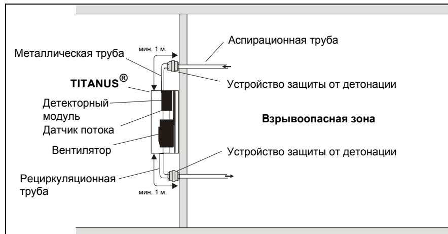
Рис. 2.21: Устройство защиты от детонации в системе забор проб воздуха и на рециркуляционной трубе.
