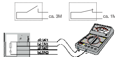
Abb.3 Prüfung der Schaltfunktion des Arbeitskontaktes (Sabotagekontakt nicht möglich)
