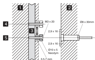
Рис.1 Расположение при лицевом монтаже макс. смещение \leq 2 мм
