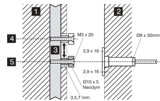
Abb.1 Stirnseitige Montageanordnung maximaler Versatz \leq 2\text{mm}
