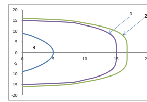
Abb.2 Abstandsdiagramm Magnet - Magnetschalter
