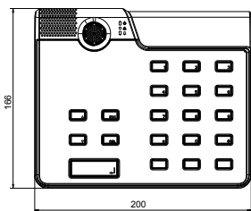
Габариты вызывной станции
