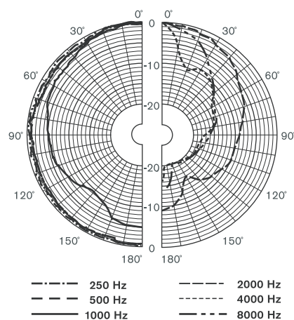
Полярная диаграмма (для розового шума)
