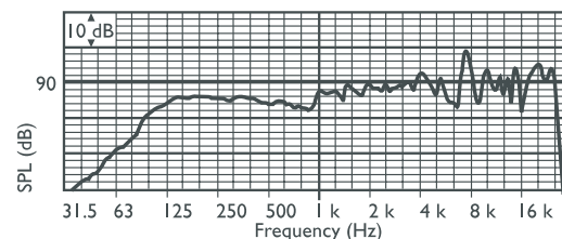
Частотная характеристика
