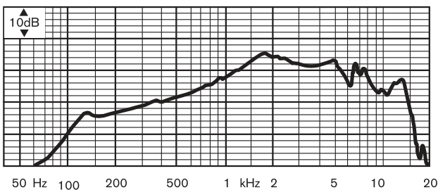
Частотная характеристика
