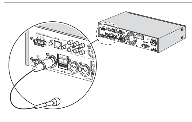
рисунок 4.1: Только разъем XLR
