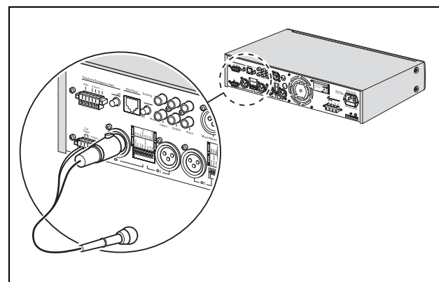
рисунок 4.2: Разъем XLR с триггером.
